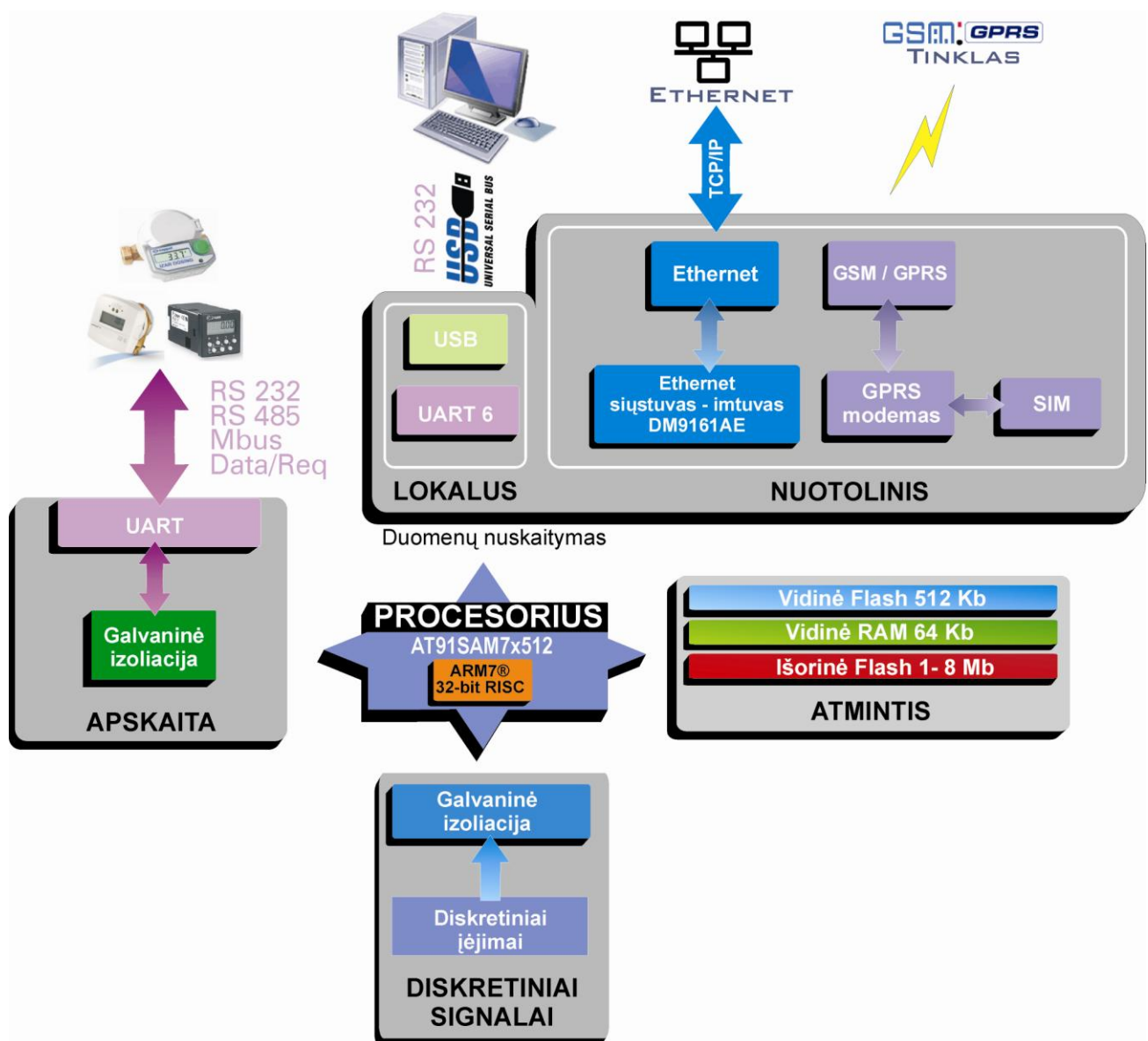
1 pav. Keitiklio MPC-333 struktūrinė schema
